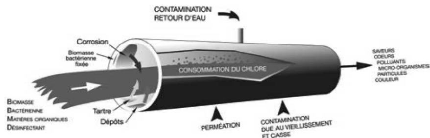
Figure 2 : Le réseau réacteur d'après Levi, 1995
