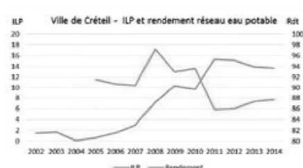
Performance réseau ville de Créteil Source Suez
