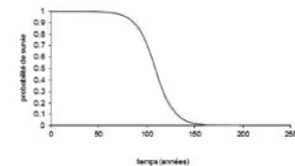
Figure 18 : Exemple de courbe de survie d'une famille de canalisations
