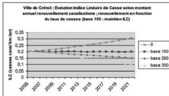
Figure 1 : Ville de Créteil – scénarii évolution taux de casses canalisations – source Suez
