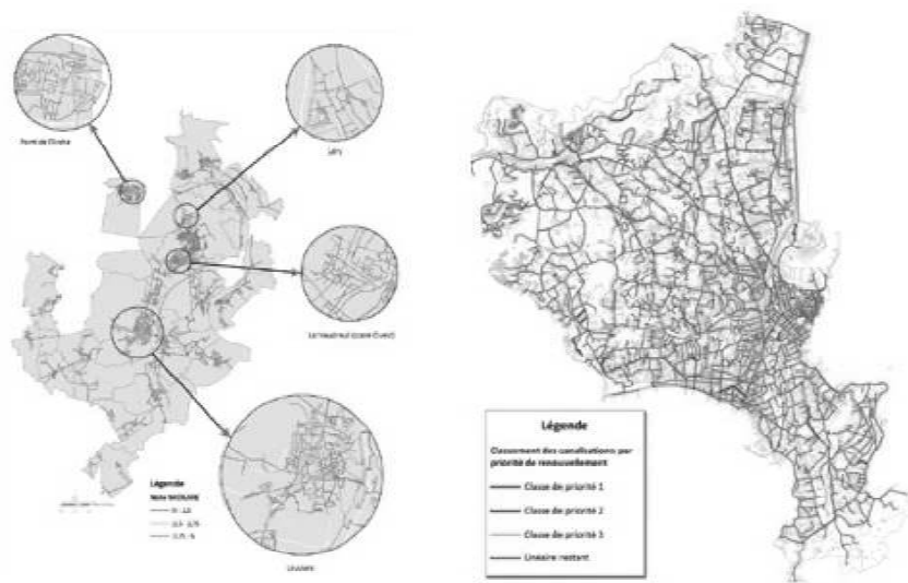
Figure 16 : Illustration de la note de risque par tronçon (Veolia) et Figure 17 – Priorité de renouvellement (SIROCCO® – G2C)
