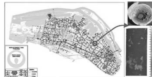
Figure 12 : Représentation de la perte d'épaisseur des conduites métalliques analysées et exemple de résultats (photographie d'une coupe transversale et répartition de l'épaisseur par profilométrie laser) – Veolia
